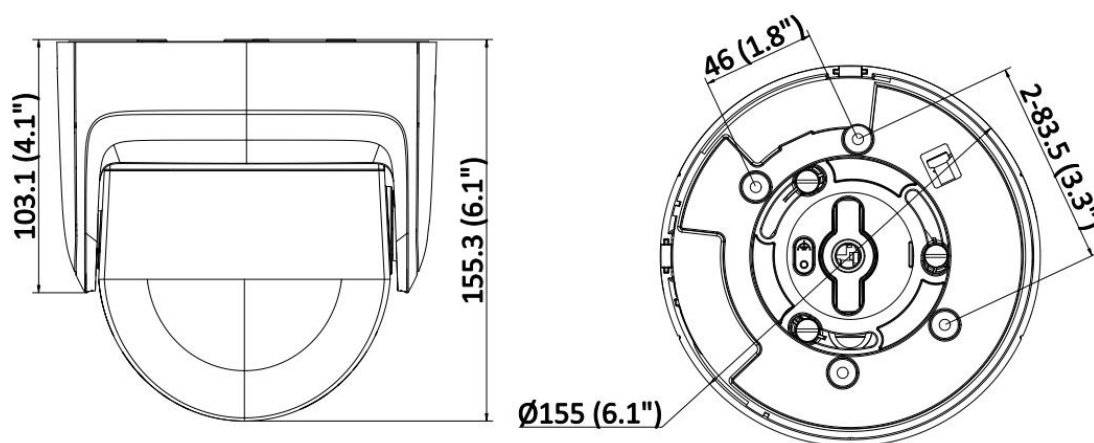
Unit:mm (inch)
